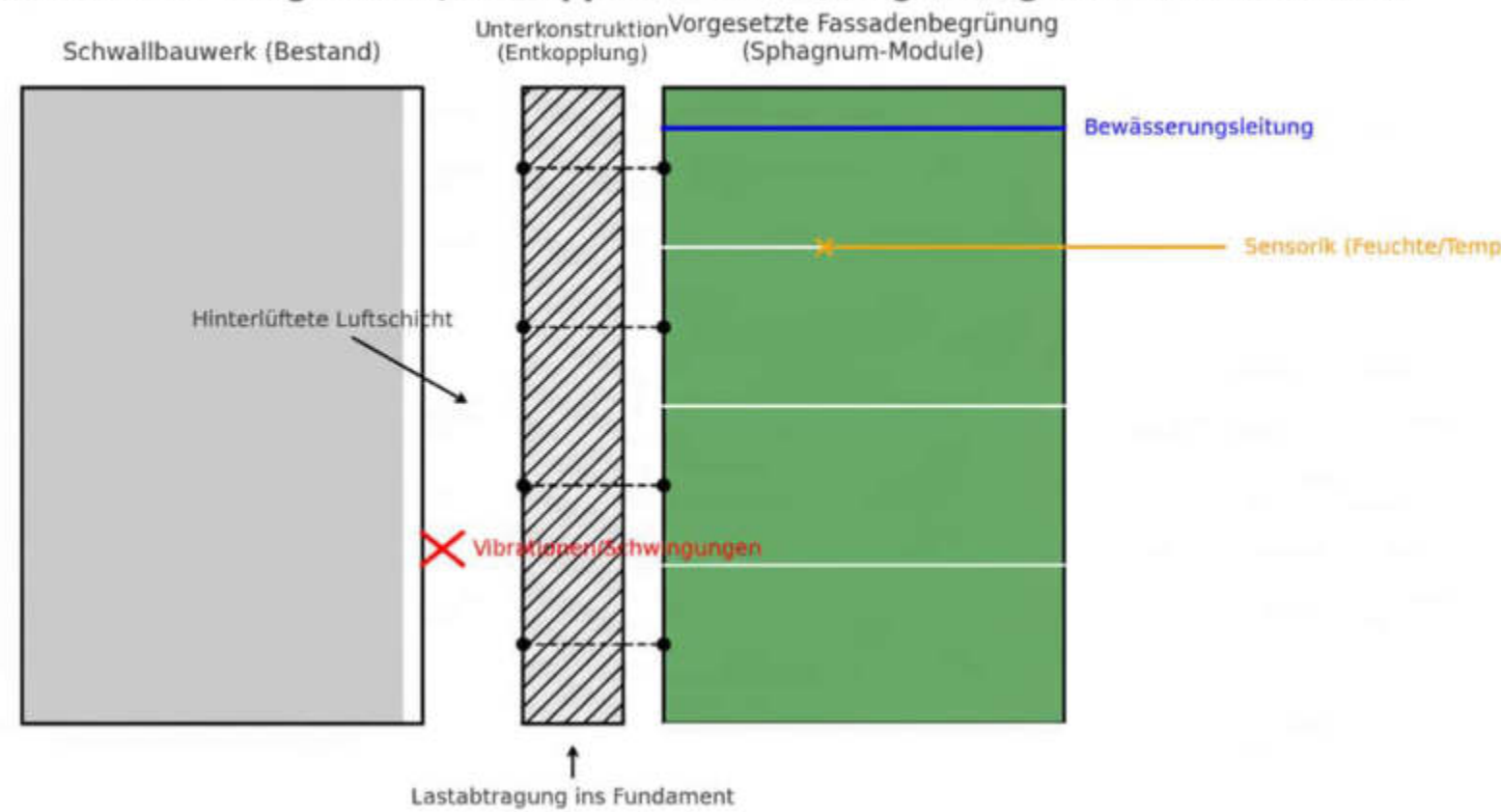
Technischer Schnitt - Vorgesetzte, entkoppelte Fassadenbegrünung am Schwallbauwerk
