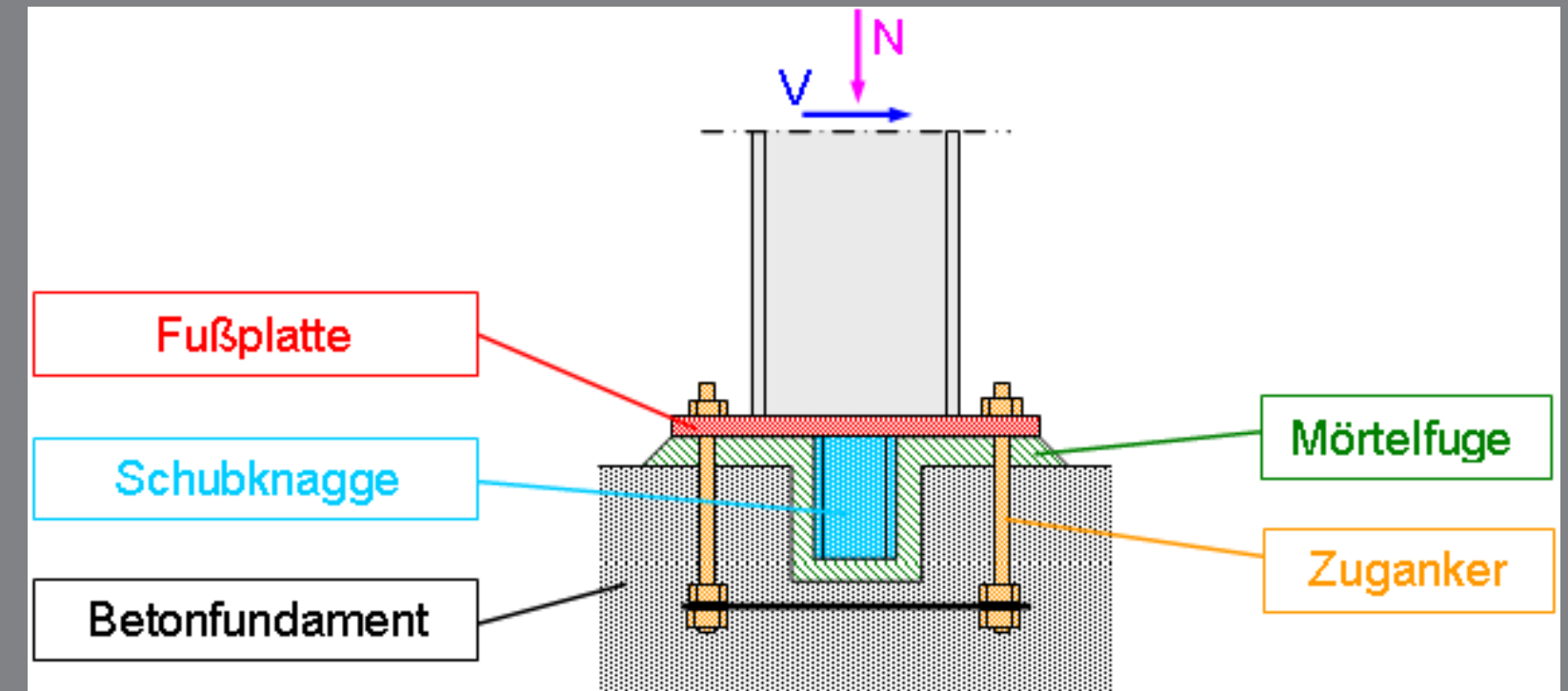
Eingespannter Stützfuß
