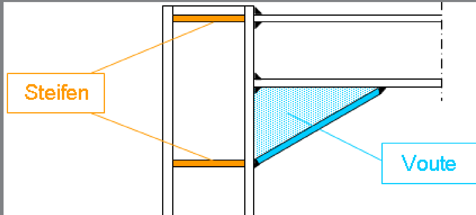
Biegesteife Ecke
