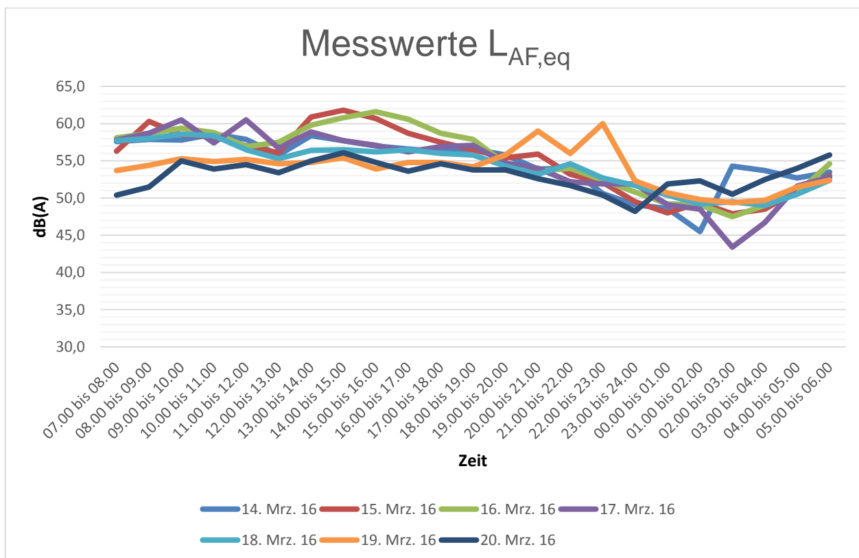
Bild 2: Pegelzeitverläufe für den Zeitraum vom 14.03.2016 bis 20.03.2016
